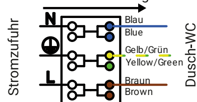
Stromanschlußdiagramm
